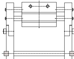
Serraggio interno. • Internal clamping. • Innenaufspannen. • Serrage interne.
